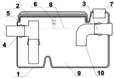
Принципиальная схема жируловителя серии СЖ "Оптима"
