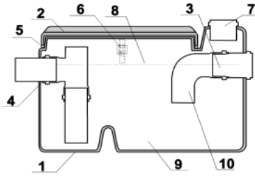
Принципова схема жируловлювача серії СЖ "Оптіма"
